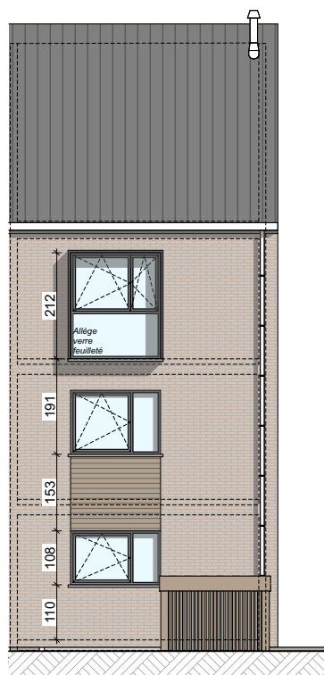
Façade avant
