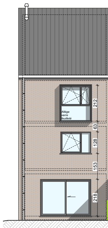
Façade arrière
