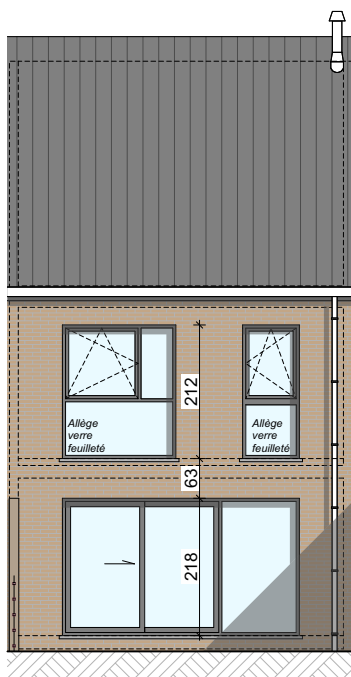
Façade arrière
