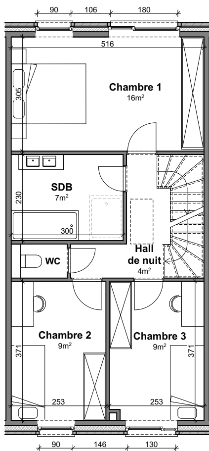
Étage
