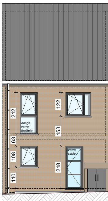
Façade avant
